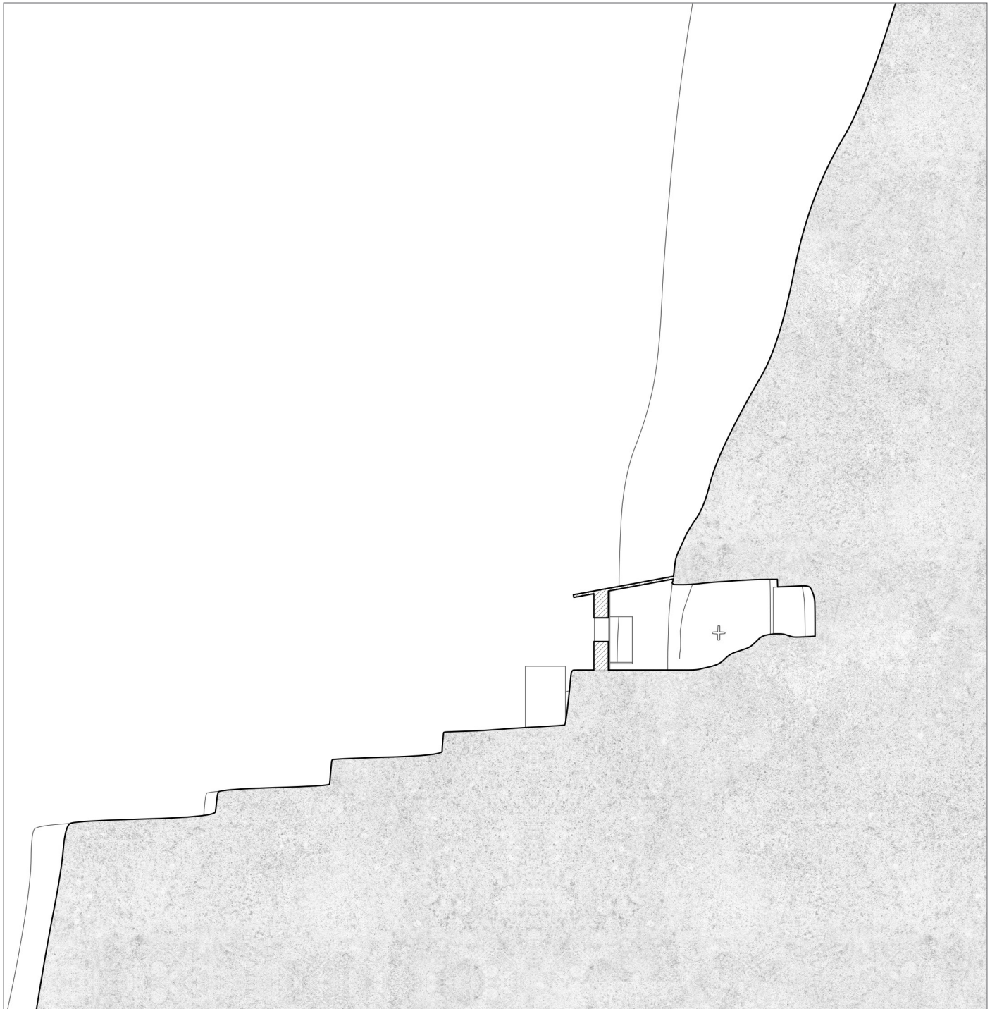
Arsema Däbrä Tiguhan Section AA (2020)
